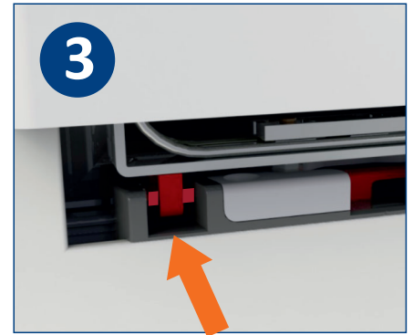
Fenster geschlossen und verriegelt. Die Pilzkopfverriegelung ist fest fixiert.
